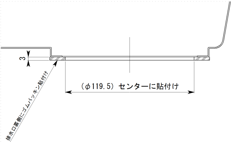
排水口部詳細
