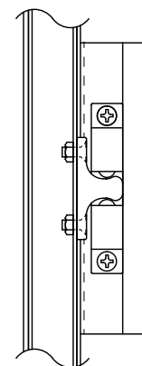
B-B' 断面
