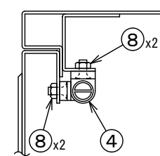
B-B' 断面
