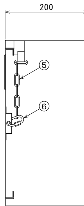
A-A' 断面
