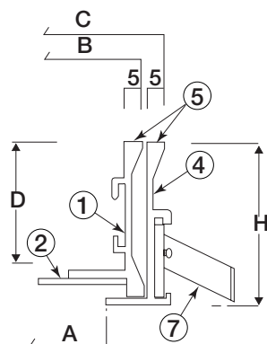
X-X' 断面詳細図
