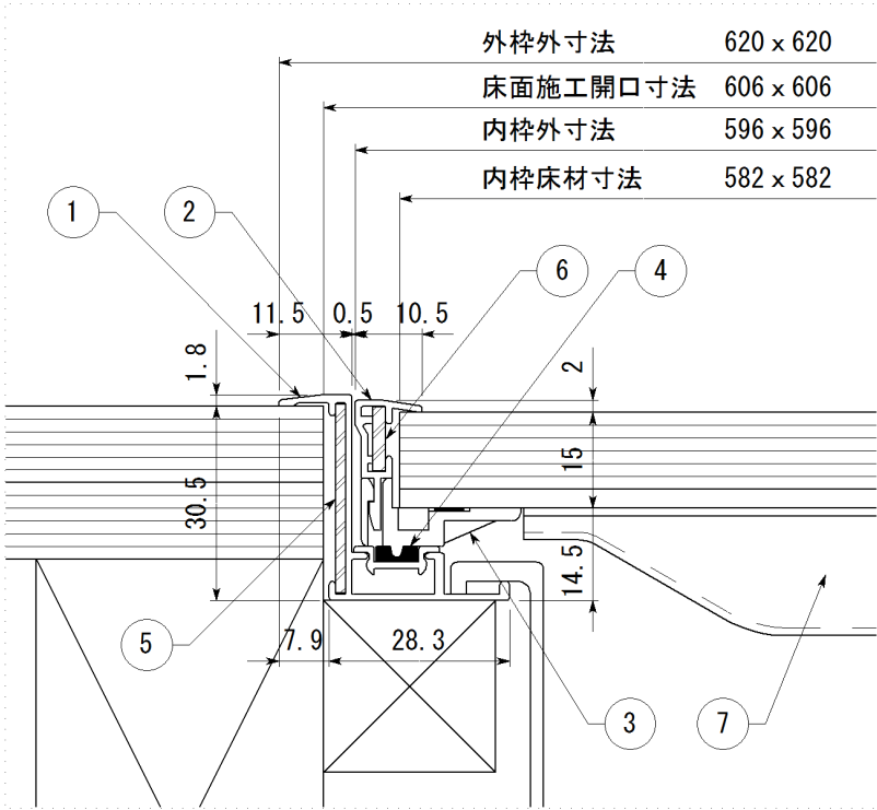
断面詳細
