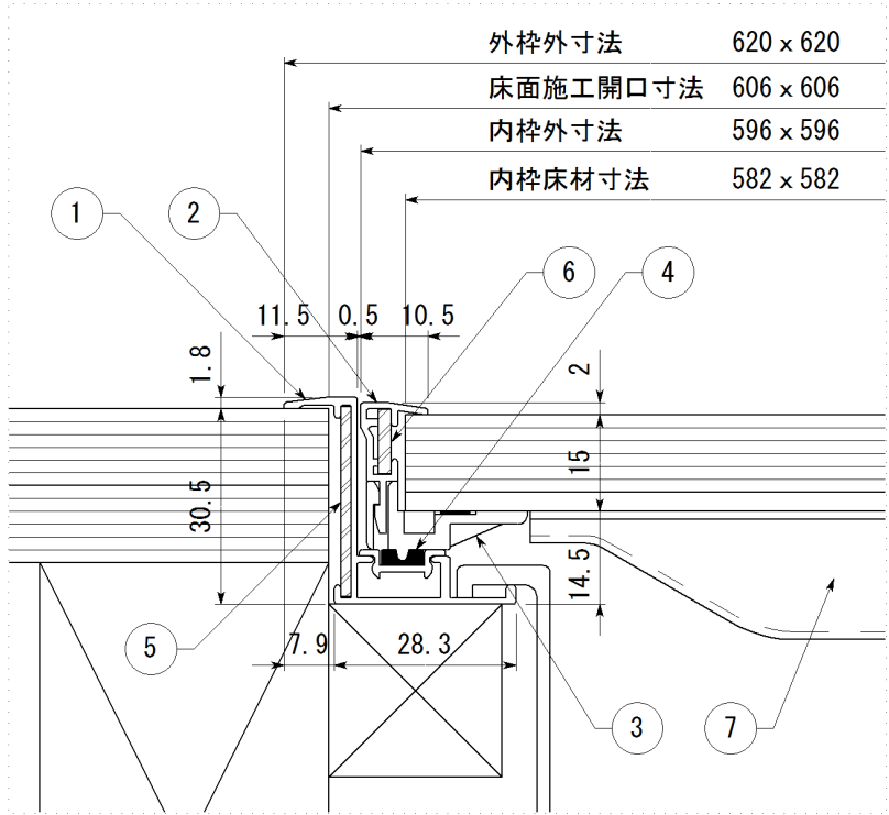
断面詳細
