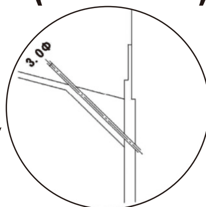
水抜き穴 詳細図 3φ穴(6か所)
